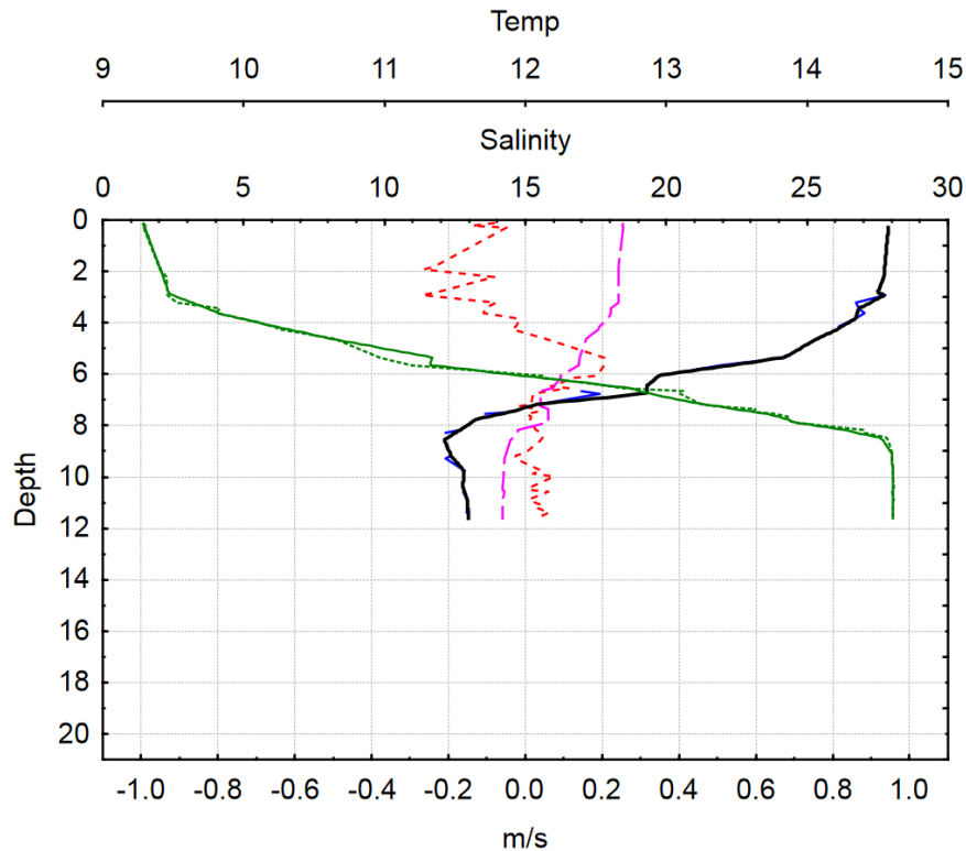
Figur 11. Profil på stasjon L1b ved nedenfor brua i Fredrikstad, hvor saltholdighet (grønn kurve), temperatur (rosa kurve), strøm i elveretningen (svart og blå kurve) og strøm på tvers av elva (rød kurve). Målingene ble foretatt 15. juni 2001 kl. 12:35-12:44 UTC.
