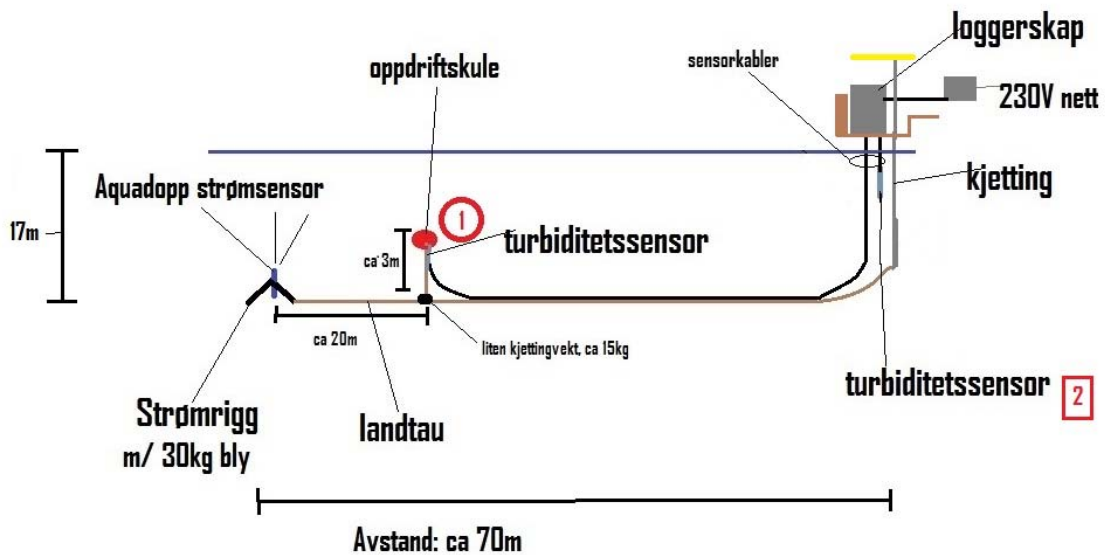
Figur 7. Oppsett av stasjon ved G1 og G2. Dyptet anvist til 17m stemmer for stasjonsoppsettet ved G1, mens det for G2 er 11m. Turbiditetssensoren merket «1» er ved posisjon G2 på ca. 1 meters dyp.
