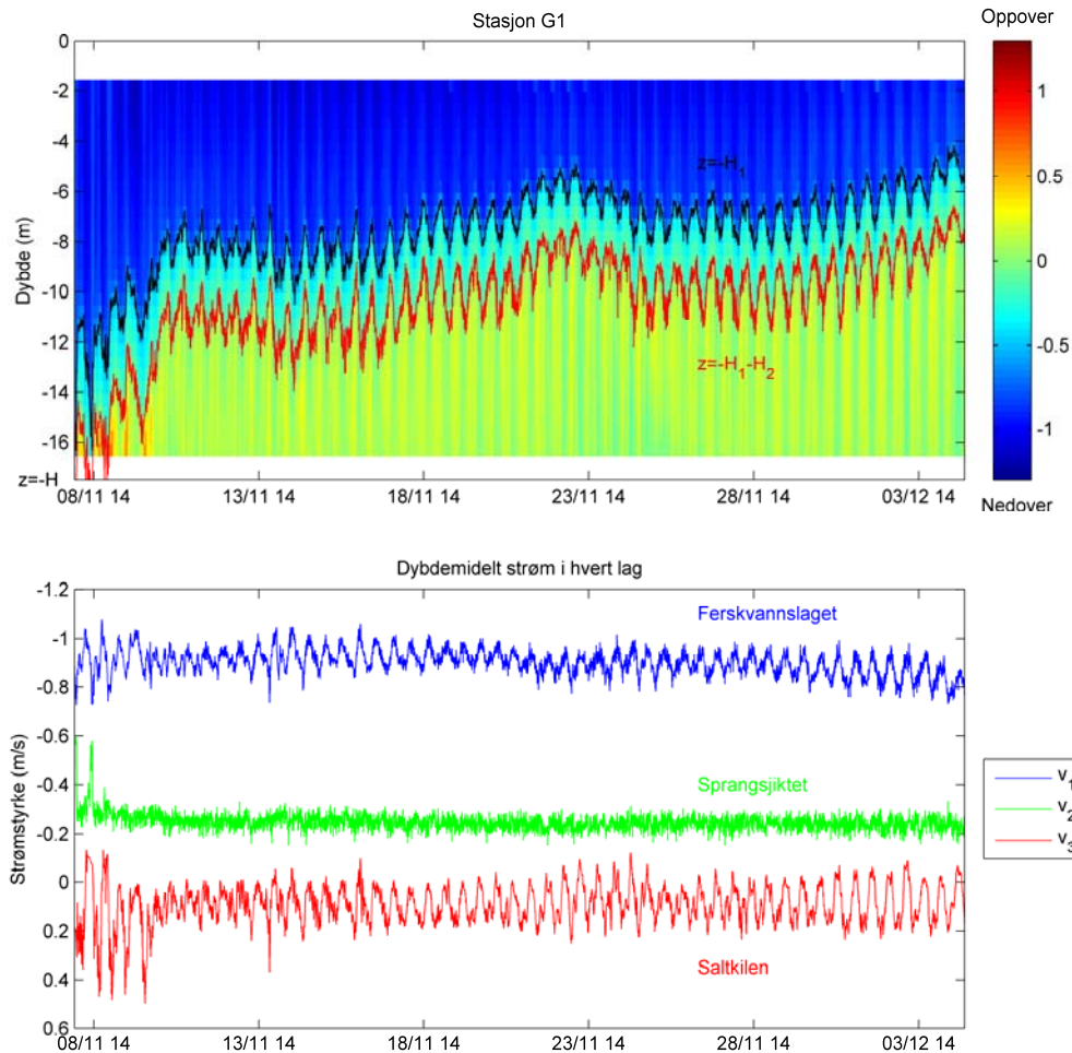
Figur 20. Øverst vises målt strøm i Glommas lengderetning på stasjon G1. Skilleflatene mellom de tre lagene er tegnet inn. Negative verdier markert med blått er strøm utover mot Hvaler, mens positive verdier er strøm oppover elva. Nederst vises den midlede strømmen i hvert lag.
