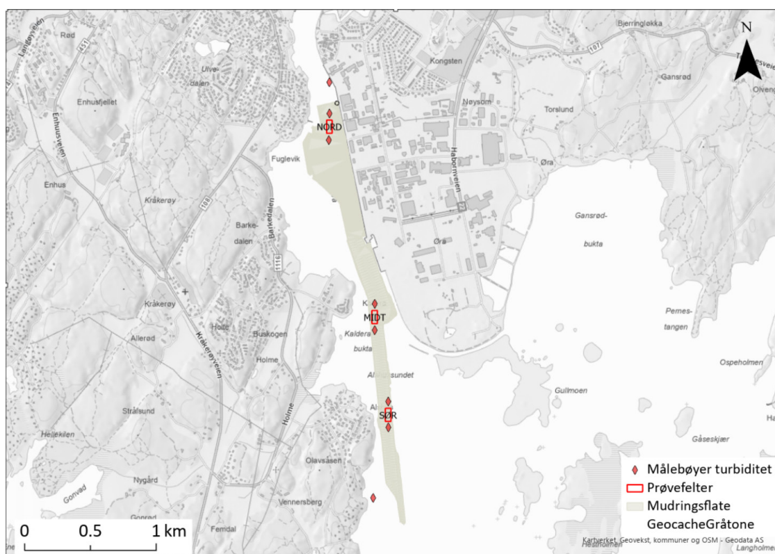
Figur 7 Prøvefelter med plassering av målebøyer for turbiditetsmålinger, samt område for plassering av referansemålestasjoner.
