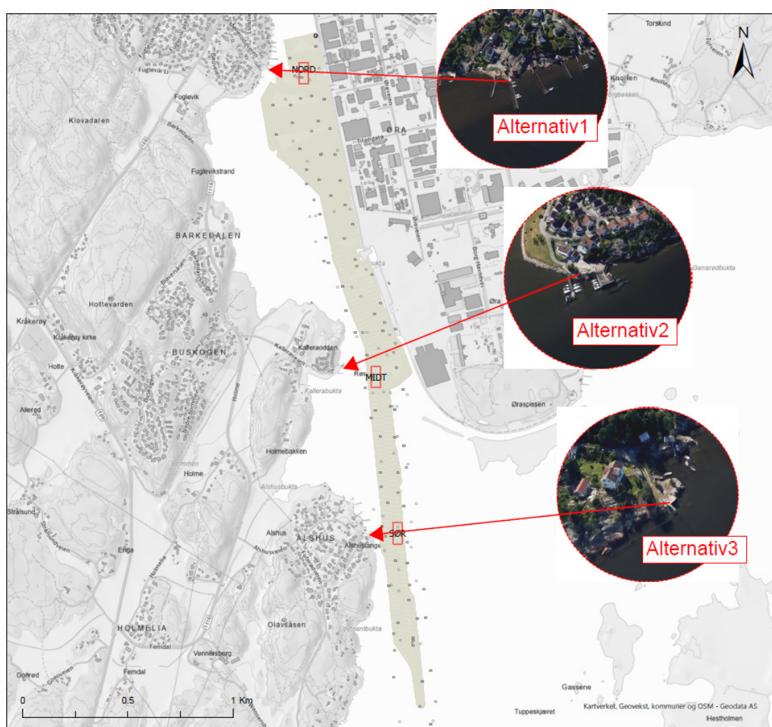
Figur 11 Aktuelle målestasjoner for støy målinger under prøvemudring.
