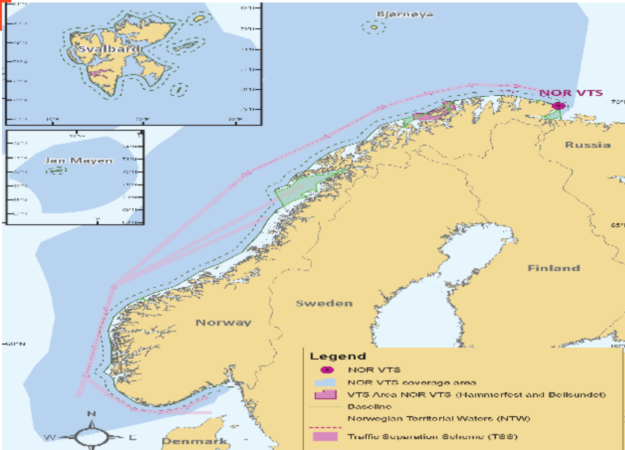
Trafikkseperasjonssystem
